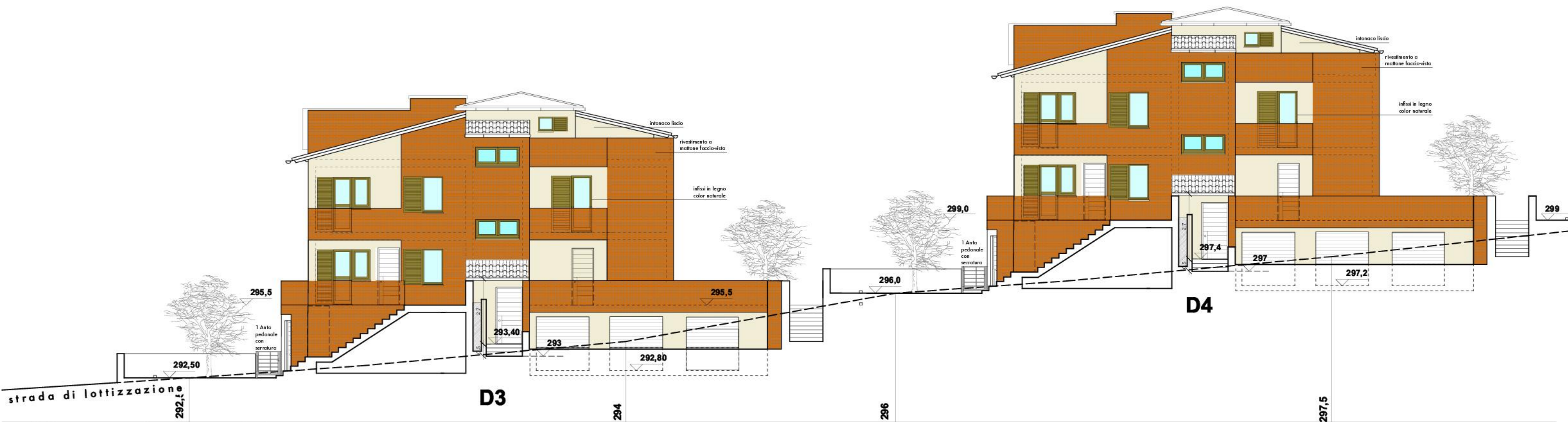
PROSPETTI NORD LATO STRADA
