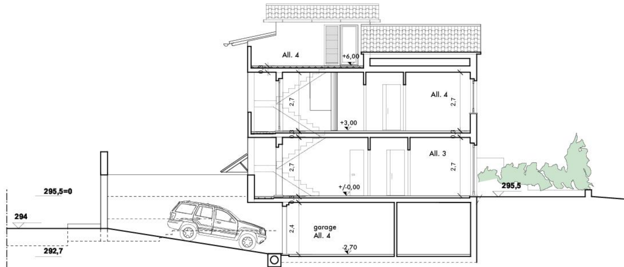
D3 SEZIONE 4 - 4'
