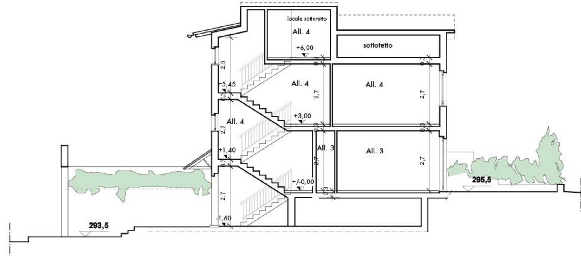
D3 SEZIONE 5 - 5'
